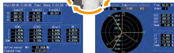
RMS values
