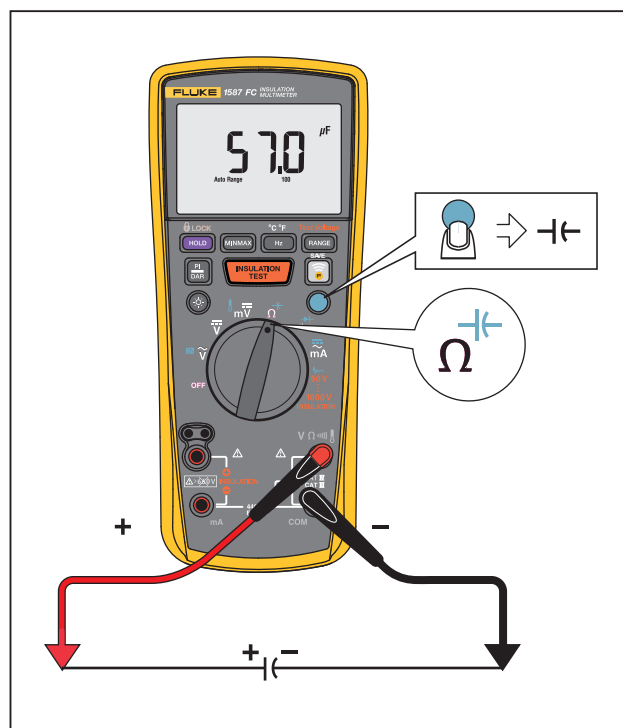
Figure 5. Mesures de capacité
