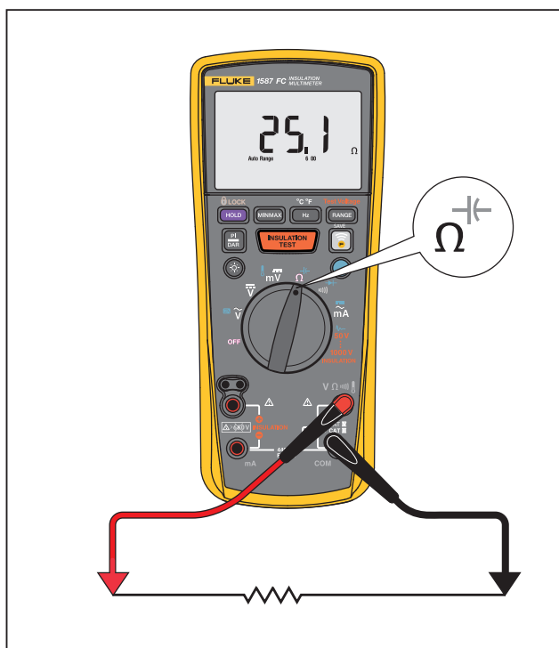
Figure 4. Mesures de résistance
