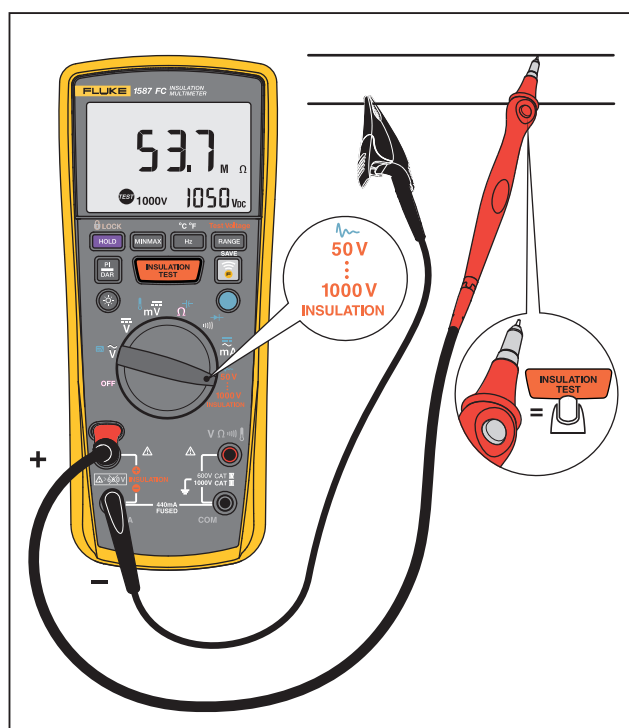
Figure 9. Tests d'isolement
