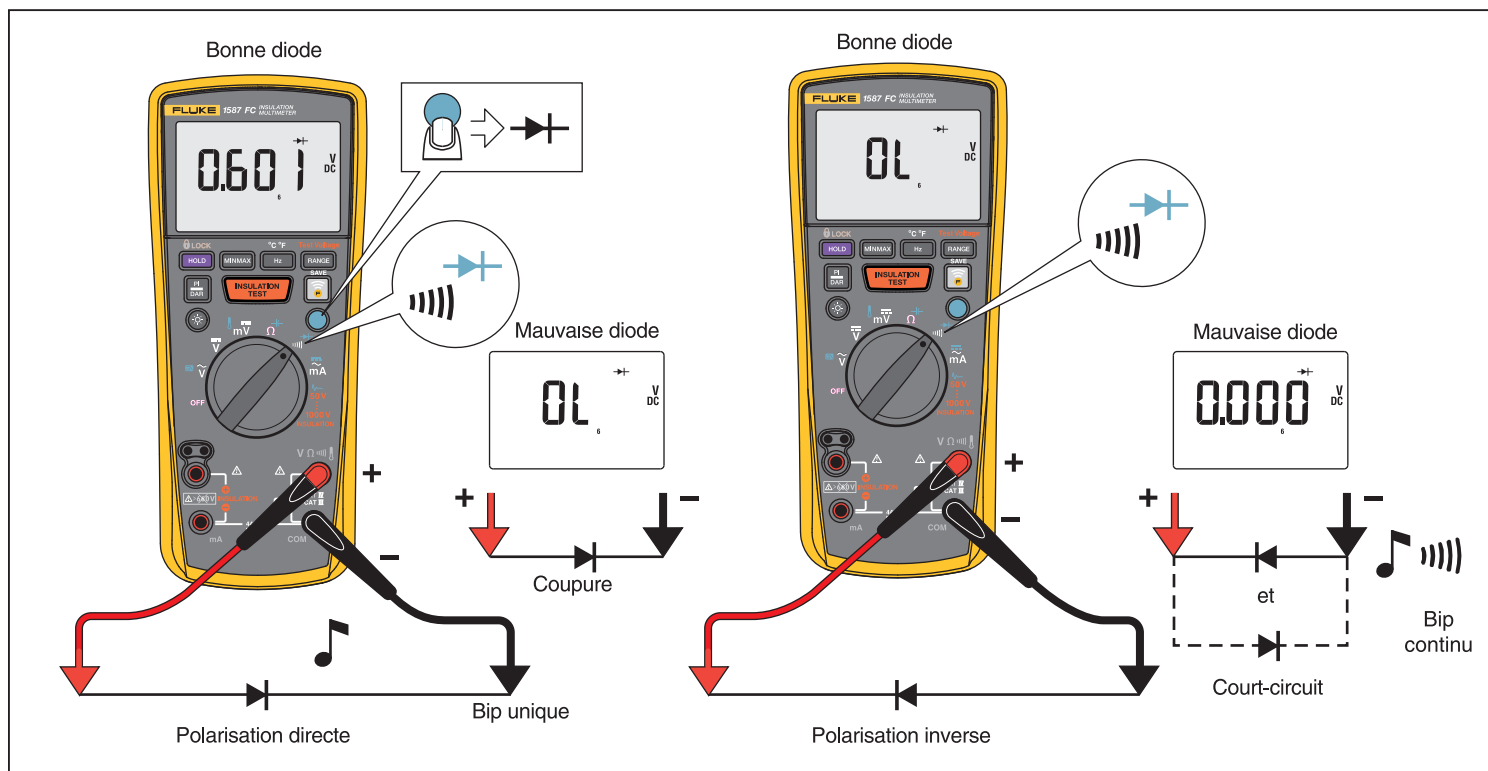
Figure 7. Contrôles de diodes
